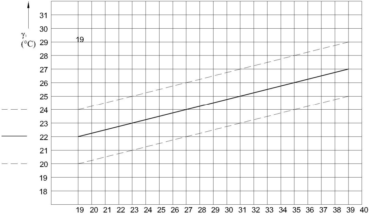
Hình B.2 – Dải nhiệt độ trong buồng lái và buồng hành khách
