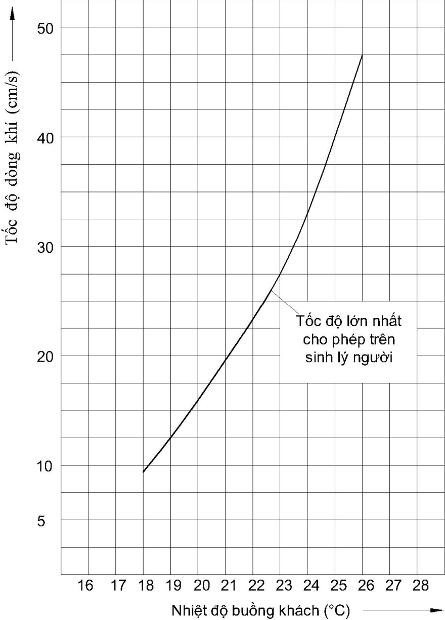
Hình B.1 – Đường biểu diễn mối quan hệ giữa nhiệt độ buồng khách và tốc độ dòng khí
