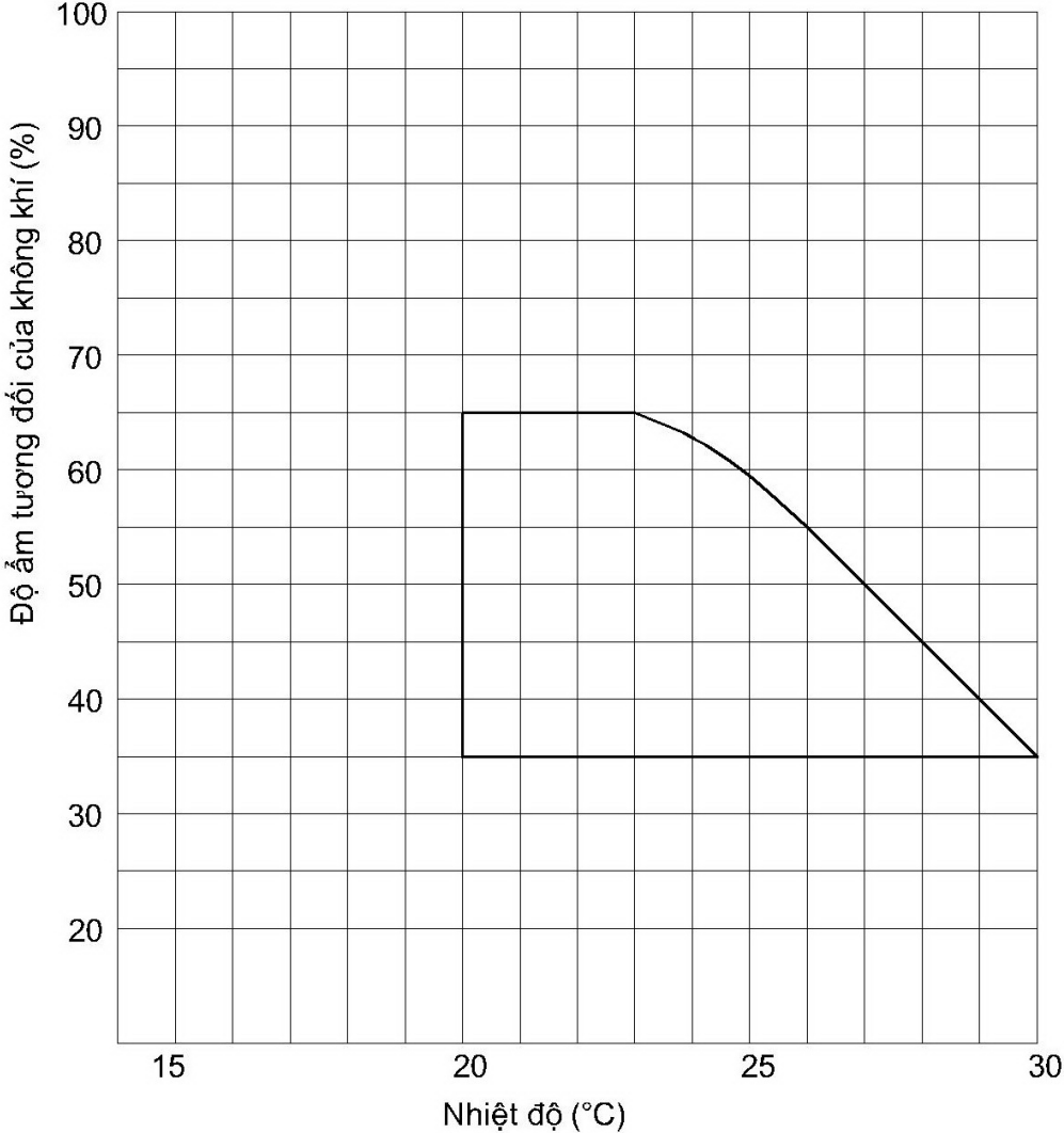
Hình B.3 – Đường biểu diễn quan hệ nhiệt độ và độ ẩm bùong khác
